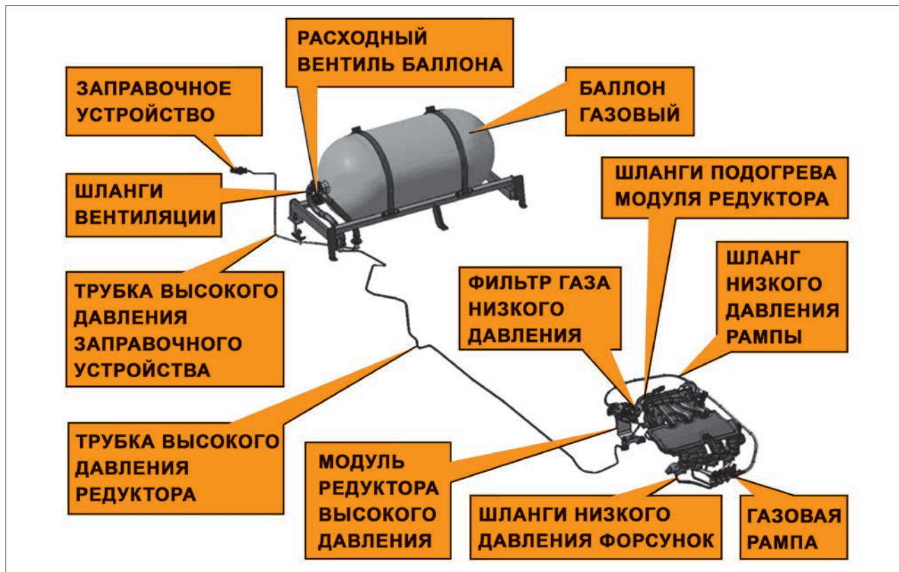
Схема соединений элементов газобаллонного оборудования в автомобиле LADA Largus CNG
